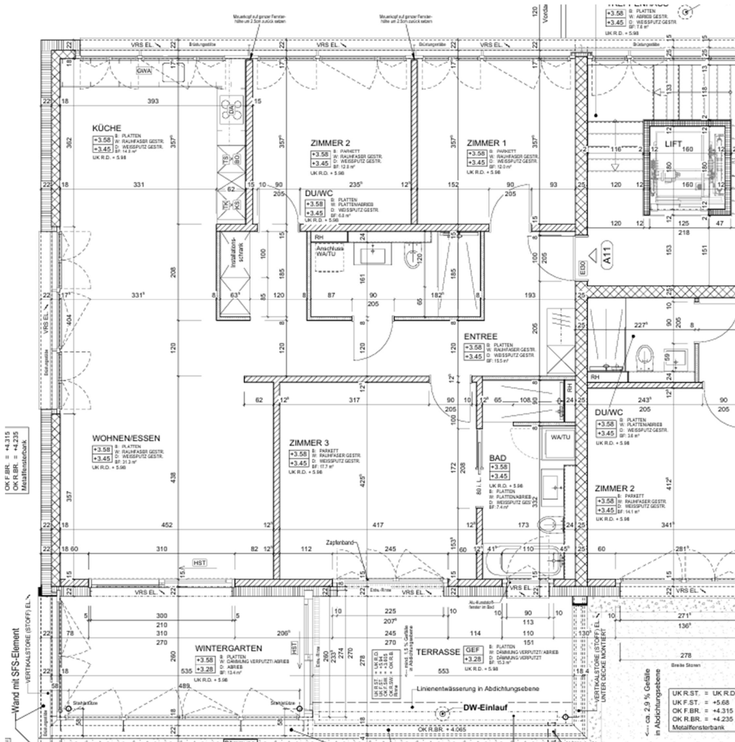
Grundriss Wohnung A1-1.2 (A11)
